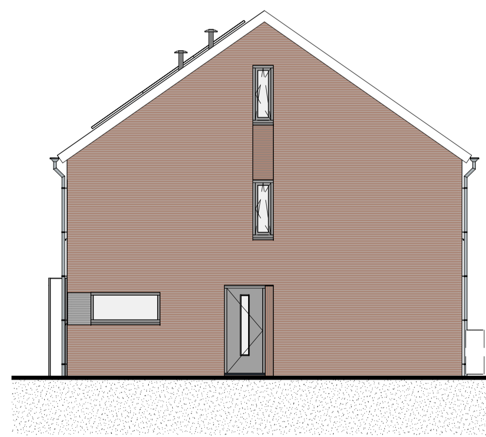
RECHTERGEVEL 1:100
