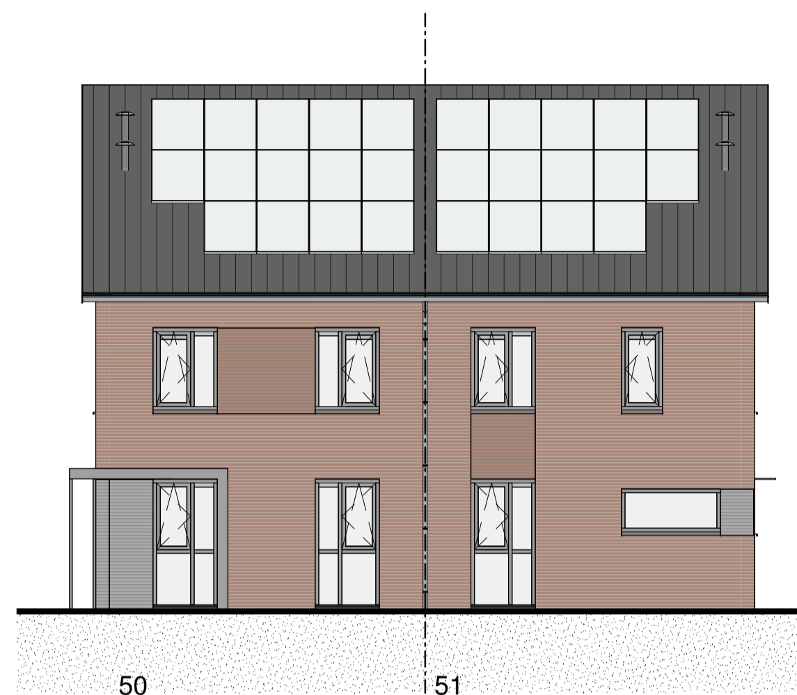
50 VOORGEVEL 1:100
